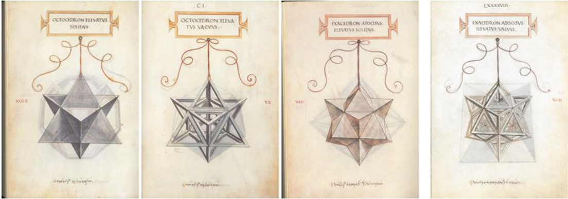
Ottaedro elevato
