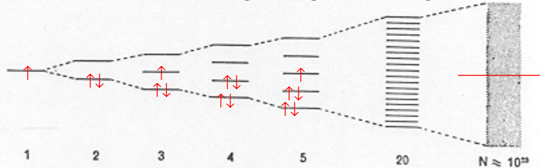
Formazione della banda di energia nel legame metallico per il litio
