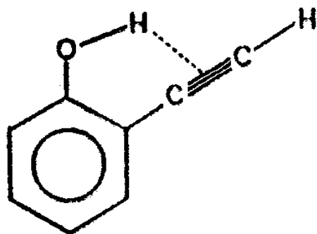
orto-idrossifenilacetilene
