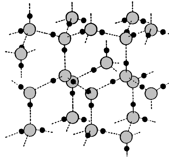
Struttura del ghiaccio
