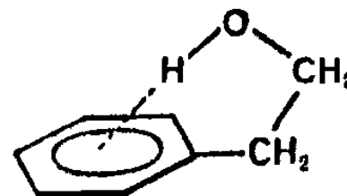
alcool feniletilico
